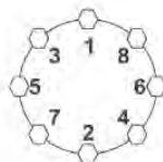
8-Lug Nuts
