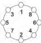
8-Lug Nuts
